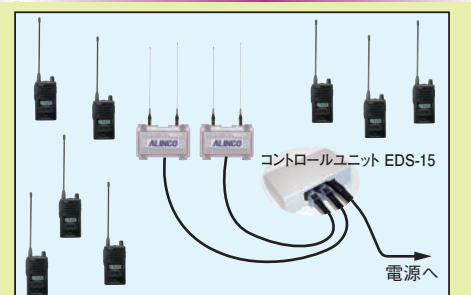
ペア接続のイメージです。DJ-M2Rでは コントロールユニットは不要です。
